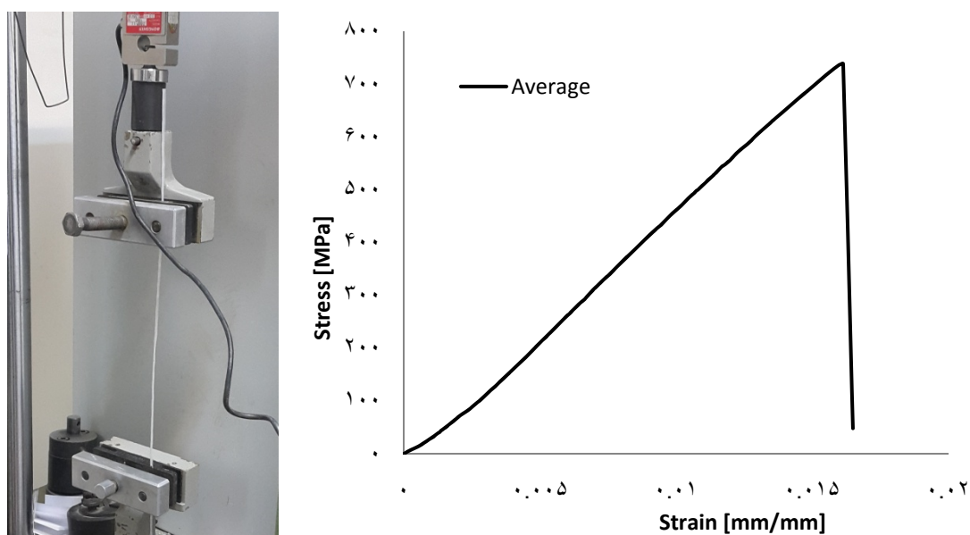
شکل (پ ۱-۱۱) رفتار کششی الیاف ARGlass
