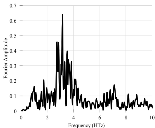
د) پاسخ فوريه سازه در راستای ۶
