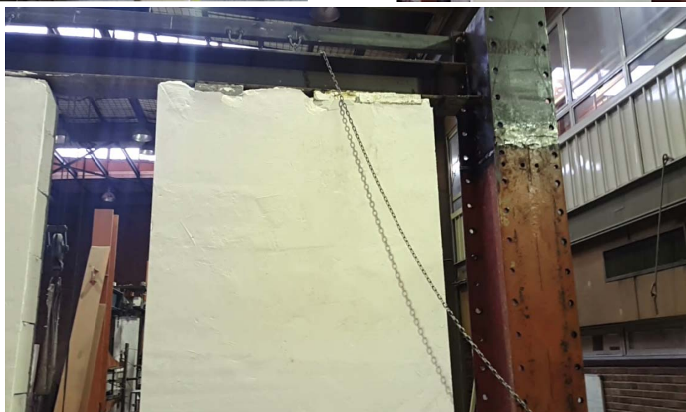
شکل (پ-۱۶) بارگذاری خمشی پانل ( ۴ نقطه ای ) بر اساس استاندارد ملی ایران
