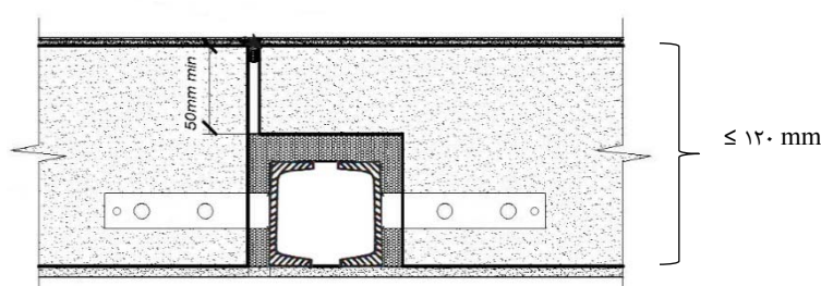
شکل (۴-۸) جزئیات اتصال دیوار به وال پست
