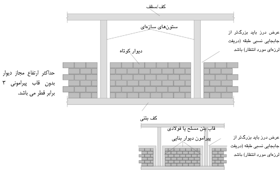
شکل (۱-۳) پارتیشن کوتاه
