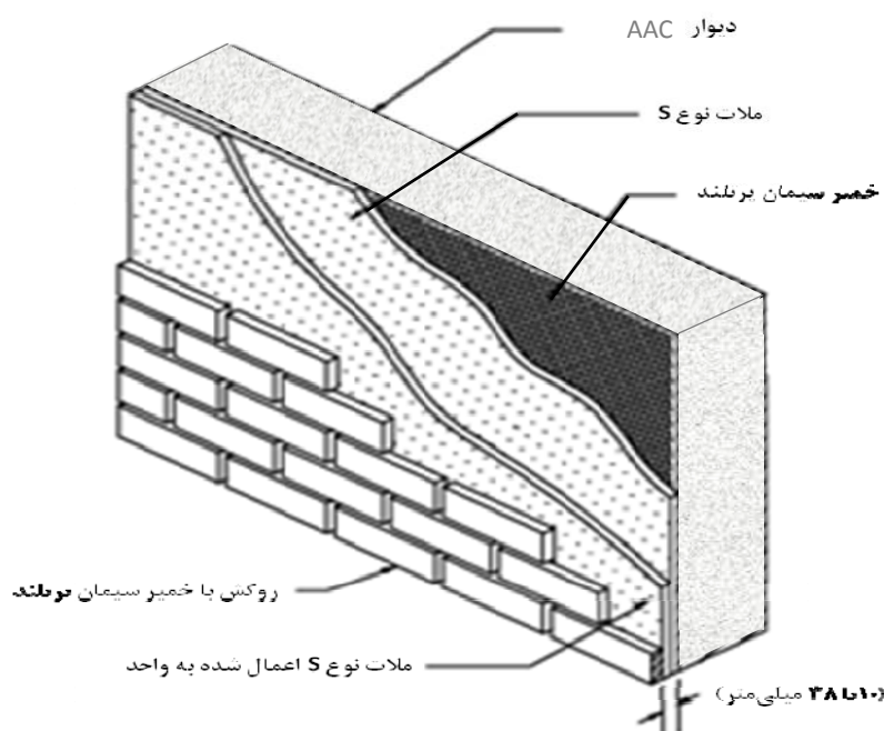
شکل ۵-۶ نمای چسبانده شده به دیوار پشتیبان AAC
