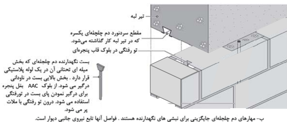
شکل ۵-۱۷ دو روش متداول برای ایجاد مقاومت در برابر بار جانبی در قسمت فوقانی دیواره های پشتیبان بلوک AAC
