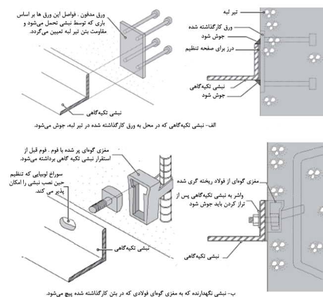
شکل ۵-۱۶ جزئیات اجرایی اتصال نبشی تکیه‌گاهی به دیوار پشتیبان
