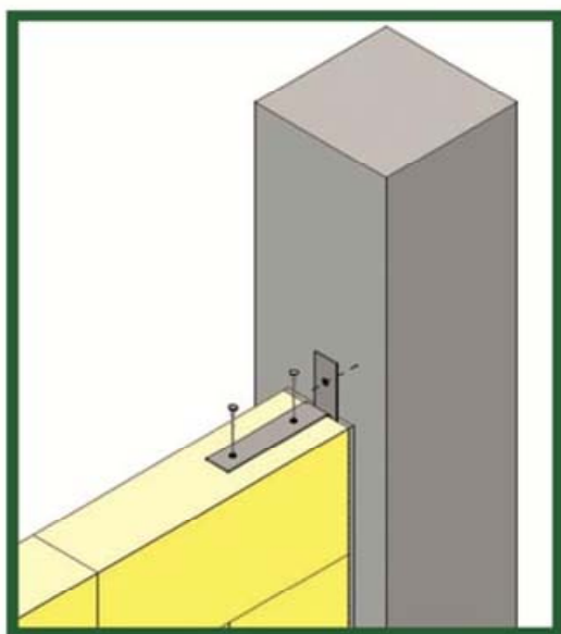
شکل (۴-۴) جزییات اتصال دیوار AAC به ستون بتن آرمه با استفاده از بست ارتجاعی
