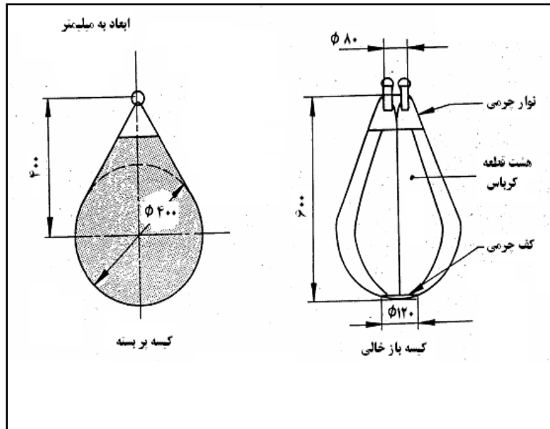
شکل (۵-۳) کیسه کروی مخروطی پنجاه کیلوگرمی
