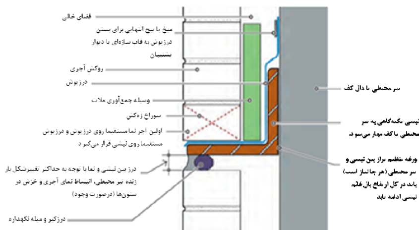
شکل ۵-۱۰ جزئیات شماتیک نشی تکیه گاهی
