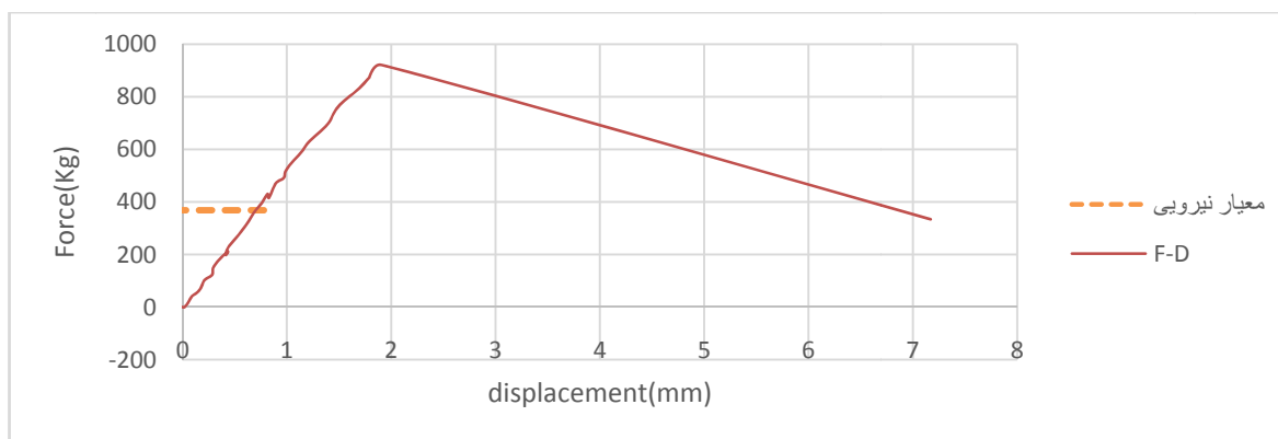
شکل (پ ۴-۲) نمودار نیرو تغییر شکل
