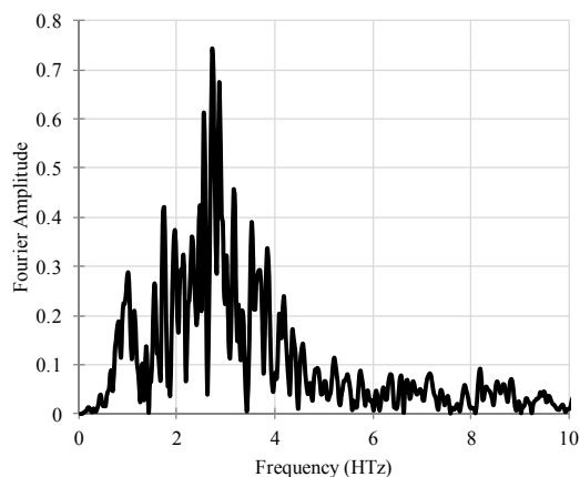
ب) پاسخ فوريه سازه در راستای ۵
