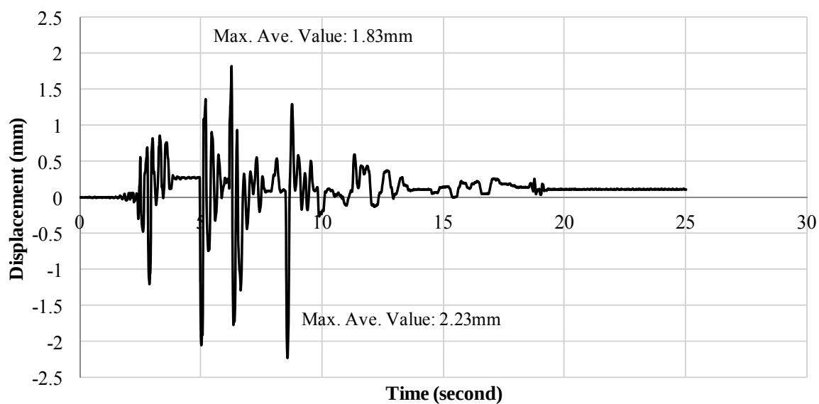
ج) دیوار شماره (۳)
