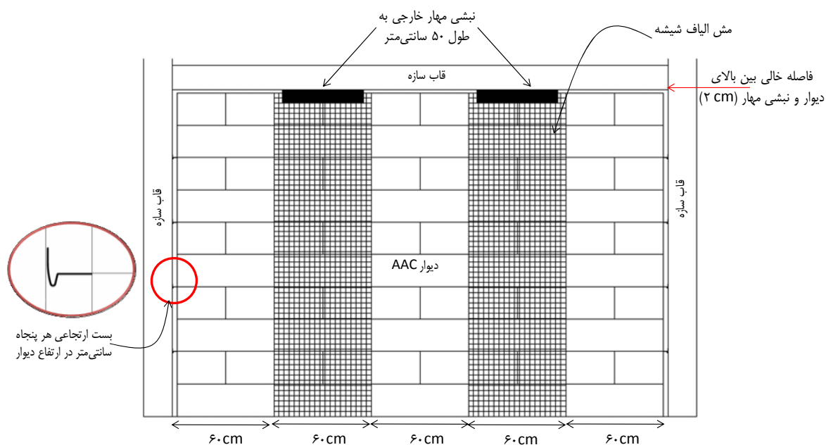
شکل (۴-۱۴) جزئیات اتصال دیوار به سقف در نمونه های تقویت شده با مش الیاف
