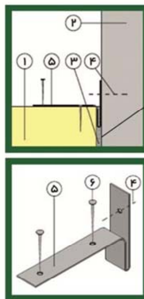
شکل (۴-۴) جزییات اتصال دیوار AAC به ستون بتن آرمه با استفاده از بست ارتجاعی
