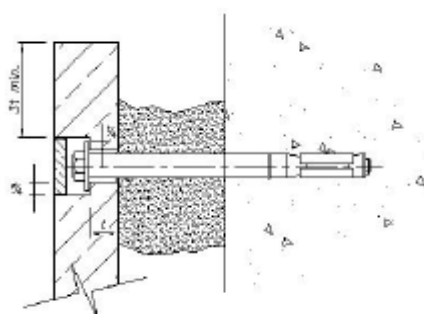
شکل ۵-۴- مهار سطحی
