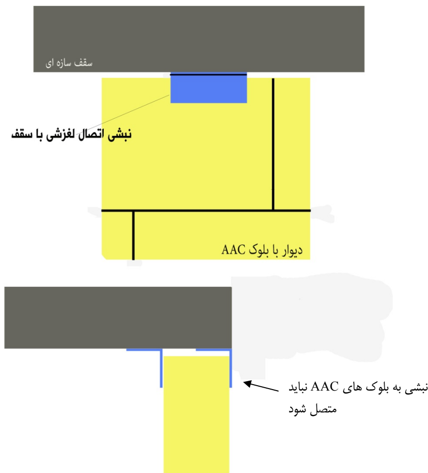
شکل (۴-۶) جزئیات اتصال کشویی دیوار خارجی از طریق نبشی به سقف سازه
