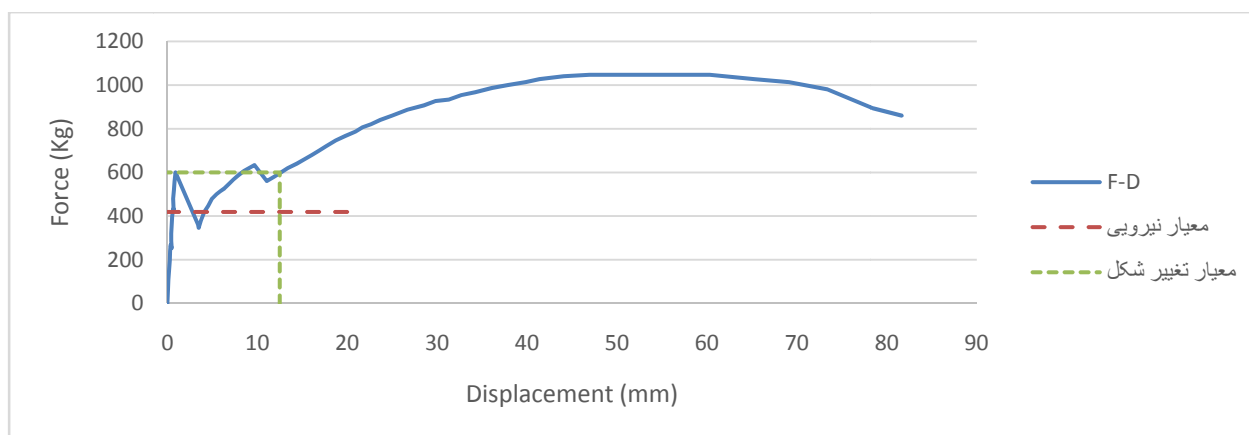
شکل (پ ۲-۱۲) نمودار نیرو تغییر شکل
