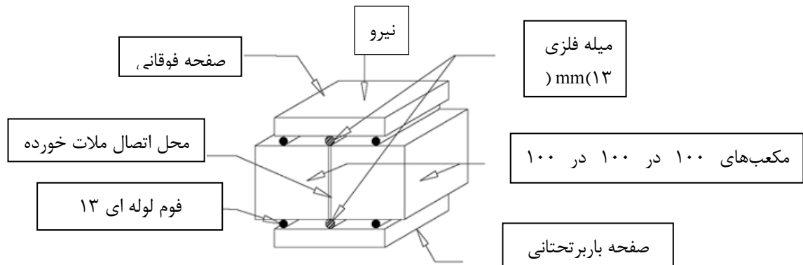
شکل (۲-۲) آزمون مقاومت گسیختگی کششی
