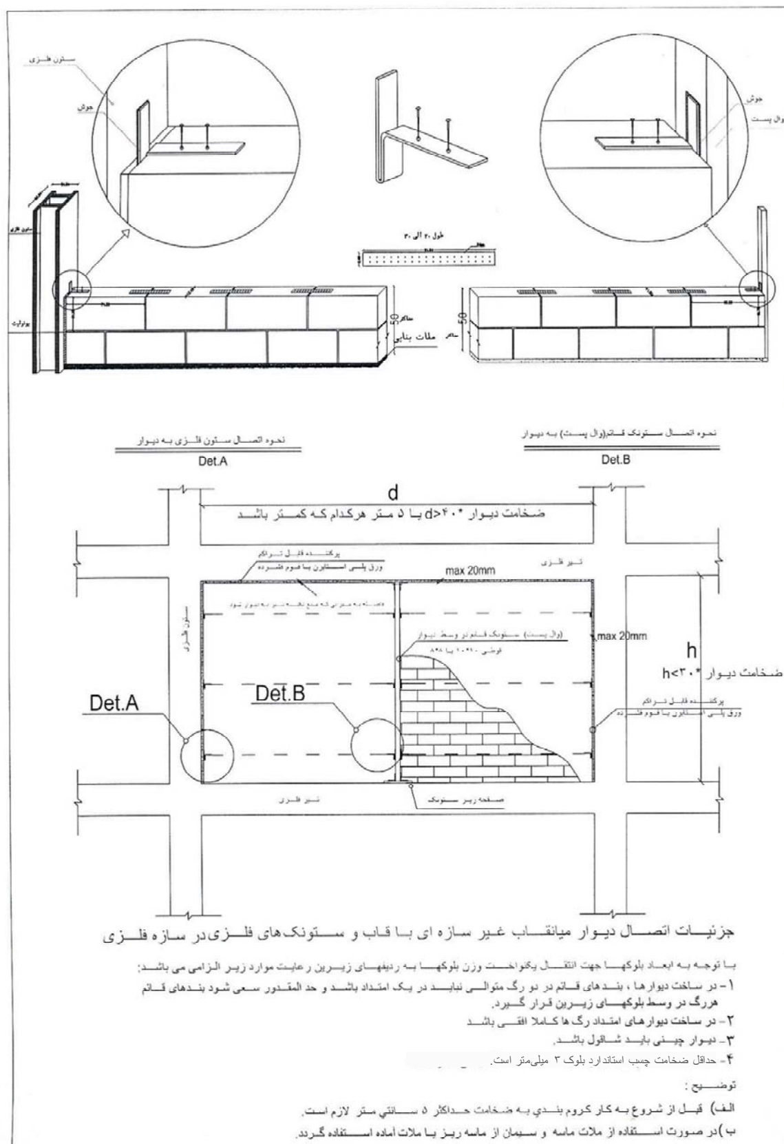
شکل (۲-۴) جزئیات اتصال دیوار AAC به ستون فلزی با استفاده از بست ارتجاعی
