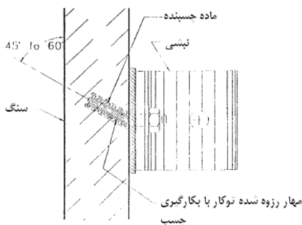
شکل ۵-۲- مهار رزوه شده توکار با بکارگیری چسب
