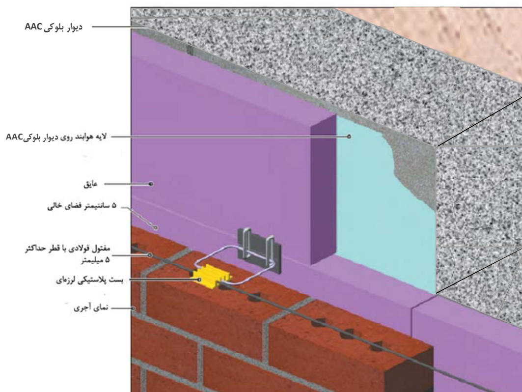
شکل ۵-۱۵ بست لرزه‌ای در نمای آجری. بست به همراه مقتول مسلح کننده در درز ملات تعبیه می‌شود
