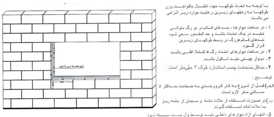
شکل (۴-۱۰) جزئیات نصب قاب پنجره بر روی دیوار AAC
