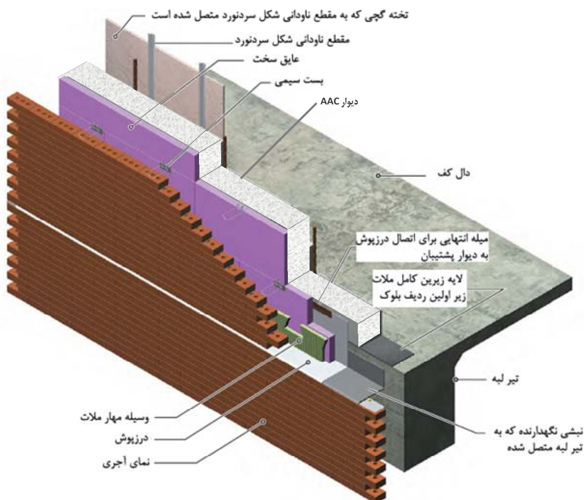
شکل ۵-۱۳ نمای بنایی آجری متصل به دیوار پشتیبان بلوک AAC
