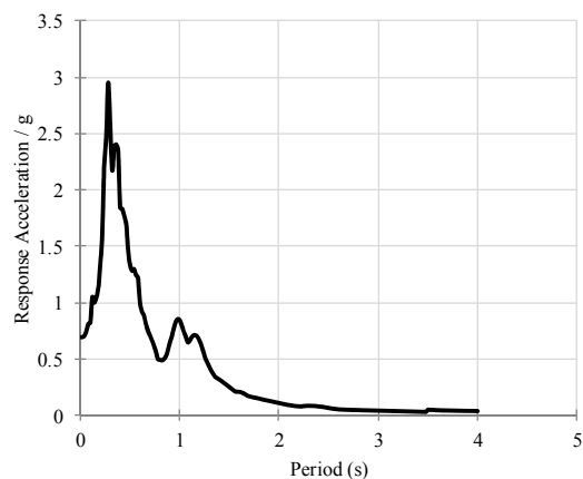
الف) طيف پاسخ سازه در راستای ۵
