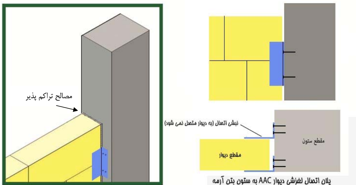
شکل (۴-۱) جزییات اتصال کشویی دیوار AAC به ستون بتن آرمه
