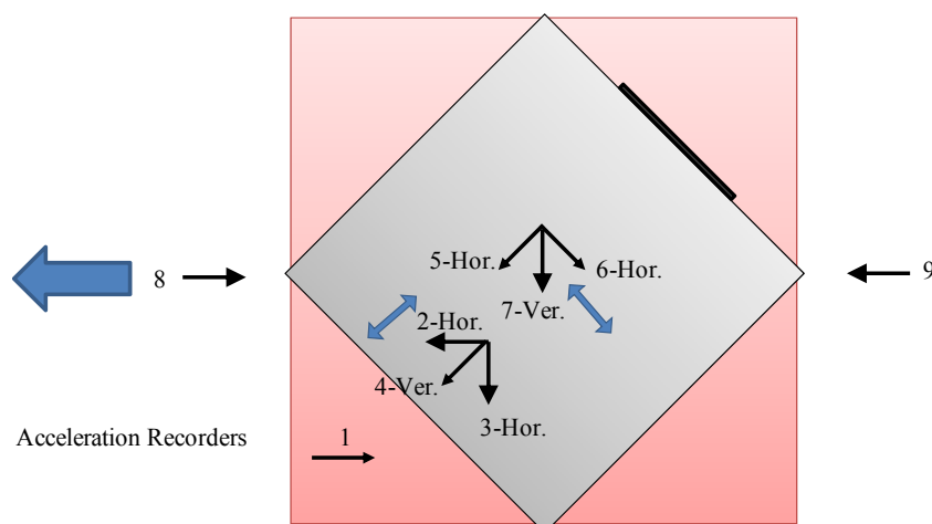
شکل (پ ۱-۲۶) کانال‌های ثبت شتاب
